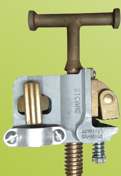
Grapa tipo "T" a Barreno Cat. FE-1132T
