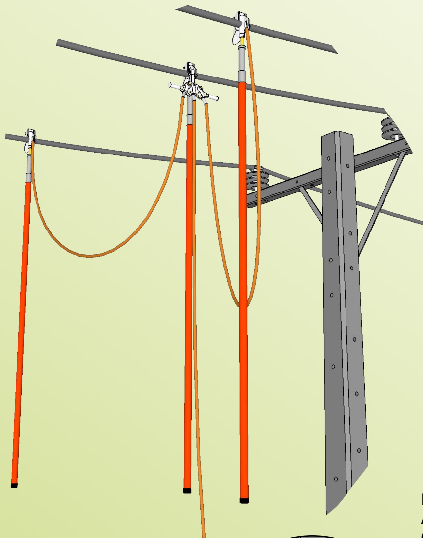
Grapa tipo "Pico Pato" Cat. FE-1192-CE
