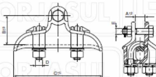
Grampo de Suspensão Monoarticulado Grapa de Suspension Pasante Single Rotation Suspension Clamp
